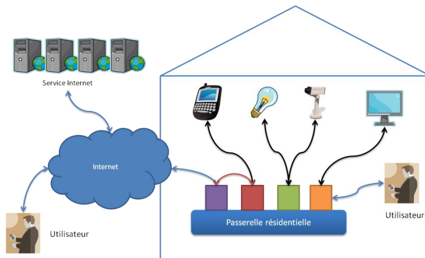
Figure 4. Passerelle résidentielle
